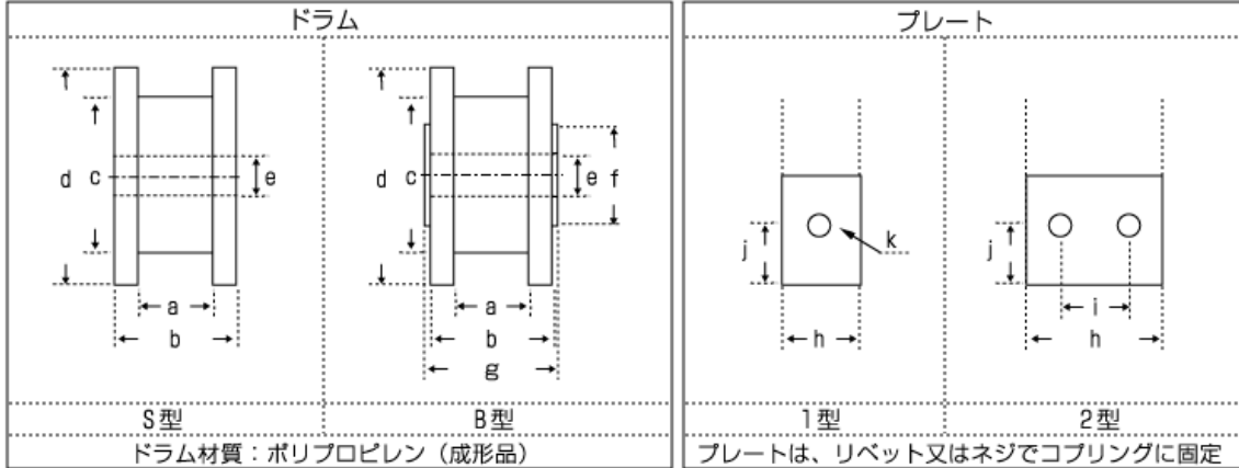
《コプリング（定荷重バネ）標準仕様、寸法一覧表》
